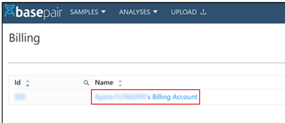
図 3 : Billing の画面
